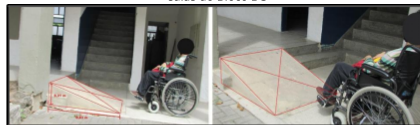
Ilustração 36–Rampa de acesso ao primeiro pavimento de salas do Bloco BC
