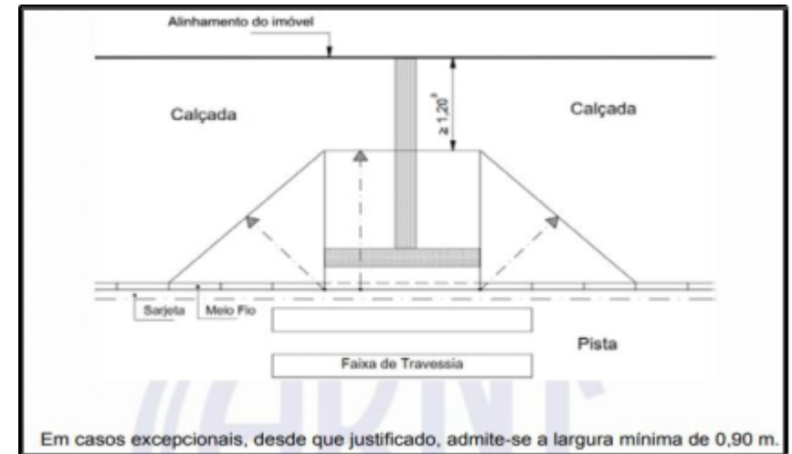
Ilustração 5-Rebaixamento de calçada – vista superior
