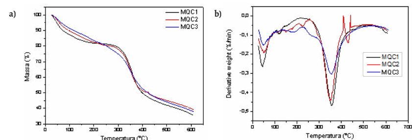
FIGURA 5 – A) CURVA TERMOGRAVIMÉTRICA (TGA) DAS MEMBRANAS DE QUITOSANA/COLÁGENO; B) SUA DERIVADA (DTG).
