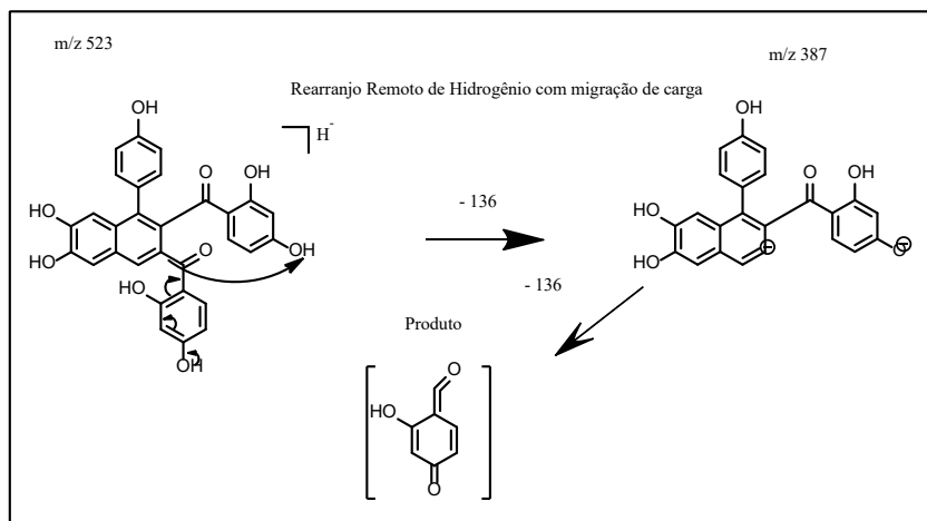
FIGURA 8 —PROPOSTA DE FRAGMENTAÇÃO DO ÍON EM M/Z 523 – URUNDEUVINA D
